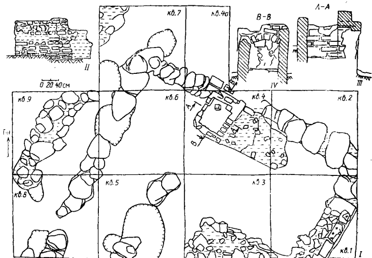
6. План раскопу рэшткаў будынка 2-й паловы 17 ст. з кафлянай печкай (раскоп 3 — 1984 г.). I — план раскопу 3; II — сістэма муроўкі тулава кафлянай печы; III — разрез А—А; IV — разрез В—В
