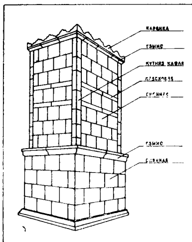
Схема размещения кафли на тулове печи.
